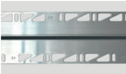
Bild 2: Dehnungsfugenprofil h=2,5 mm mit breiten Auflage-schenkeln und schwarzer Silikoneinlage / Image 2: Expansion joint profile h=2.5 mm with wide support legs with black silicone insert
