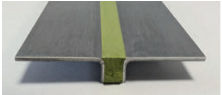
Bild 5: Dehnungsfugenprofil für nachträglichen Einbau, individuellen Schenkelbreiten und Farben / Image 4: Expansion joint profile for retrofitting, custom leg widths and colours
