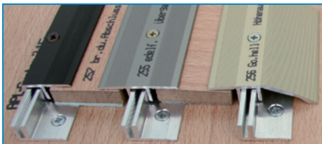
Beispiel: APL-System 7 - 15 mm (siehe Seite 95 - 98) example: APL-system 7 - 15 mm (see page 95 - 98)
